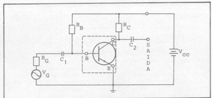
Figura 1 - Amplificador de tensão do tipo Emissor Comum
